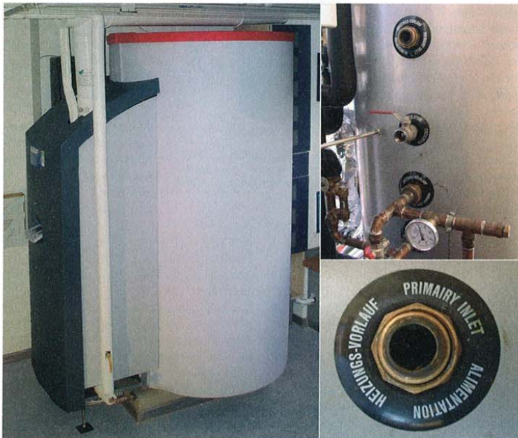
Bild 2 Kompakte solare Kombianlage der Firma Solvis (l.) und Energiespeicher der Firma Austria Email mit bereits angebrachter Wärmedämmung (o.) und genau gekennzeichneten Anschlüssen (u.)
