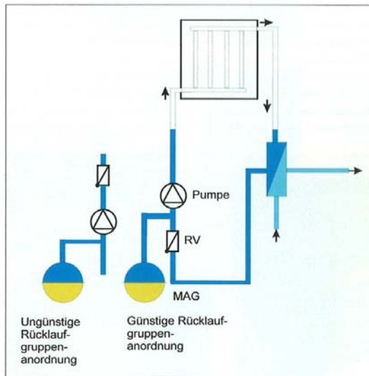
Abbildung 3: Das Stagnationsverhalten hängt von der Position der Rückschlagklappe ab (Quelle: AEE INTEC)
