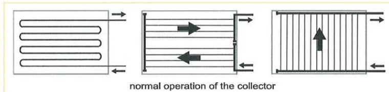
Bild 6 Hydraulische Kollektorverschaltung mit gutem Entleerungsverhalten (Quelle: AEE Intec)
