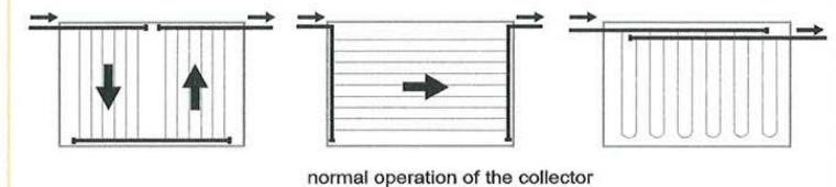
Bild 7 Hydraulische Kollektorverschaltung mit schlechtem Entleerungsverhalten (Quelle: AEE Intec)
